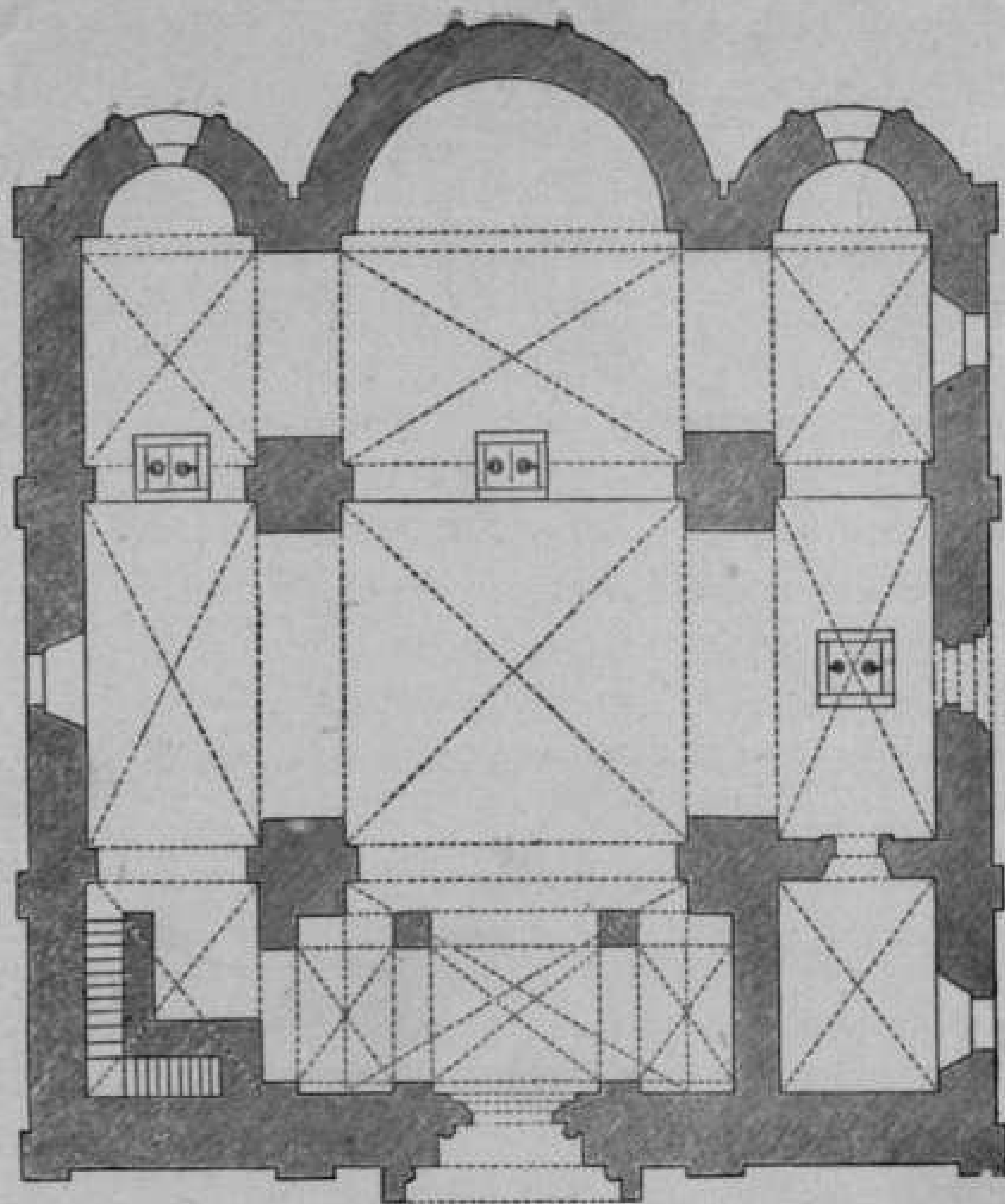
Планъ церкви св. Станислава.
