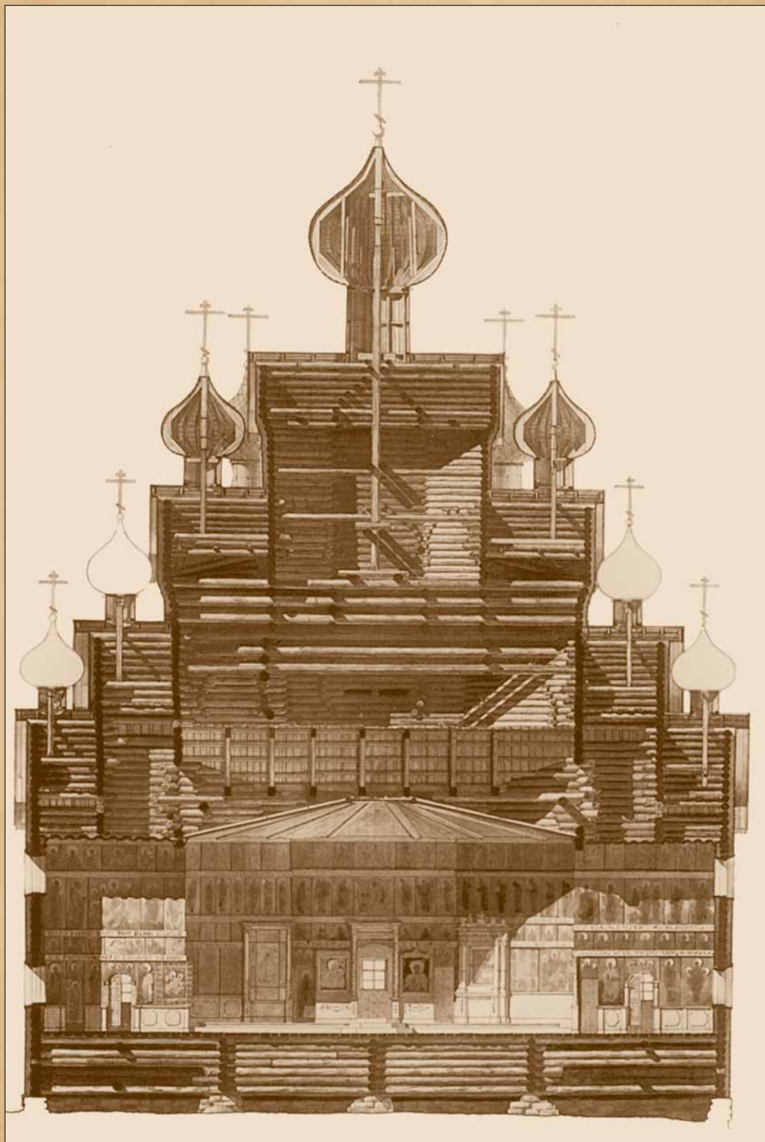
Покровская церковь близ Вытегры. Реконструкция. Разрез
