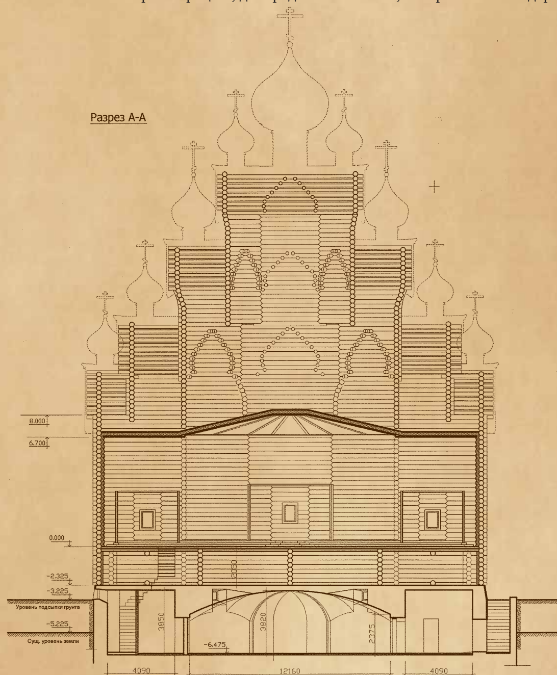
Проект реставрации церкви Покрова Пресвятой Богородицы. Фрагмент документации
